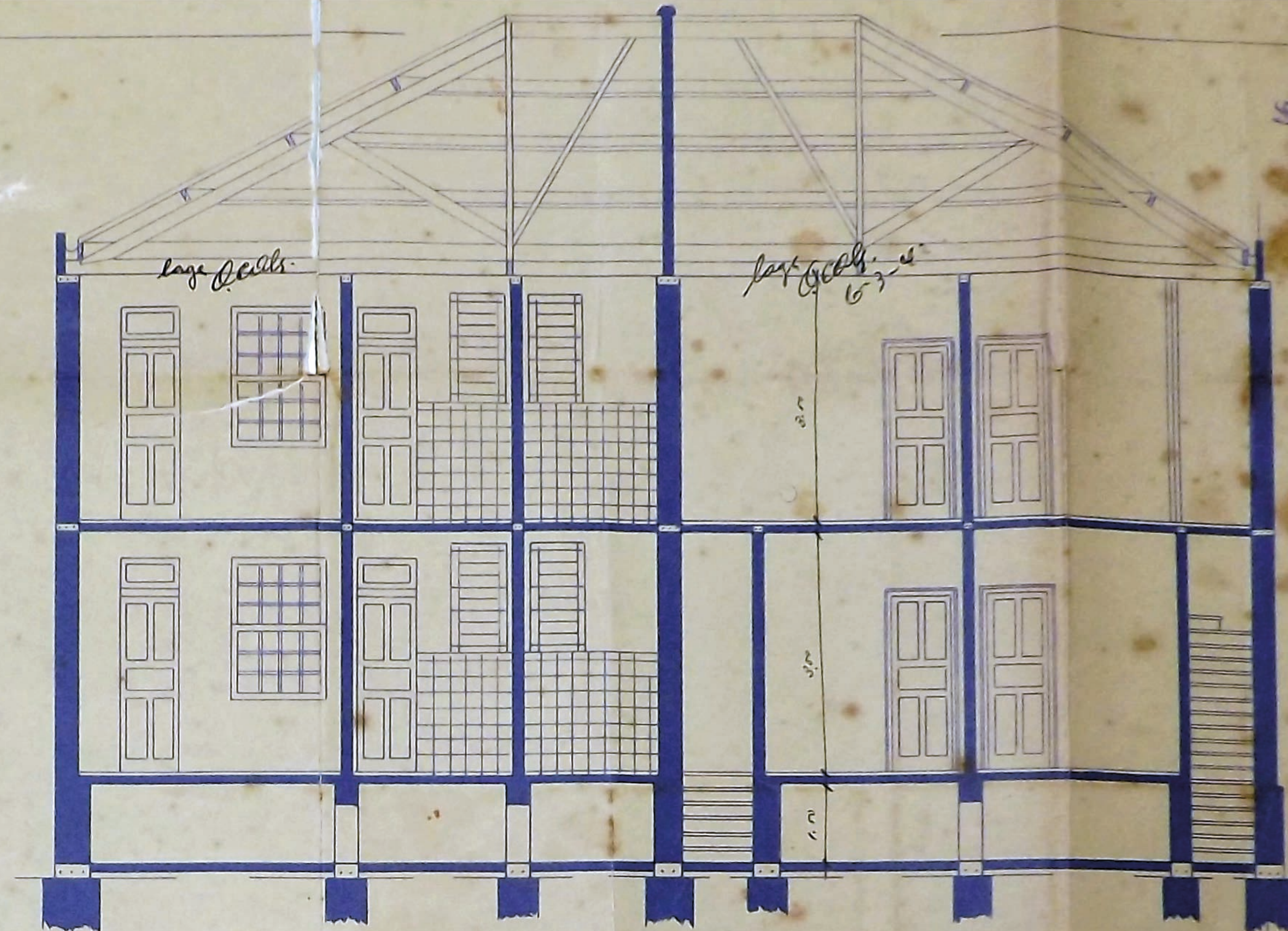
SECÇÃO AB-1:50
