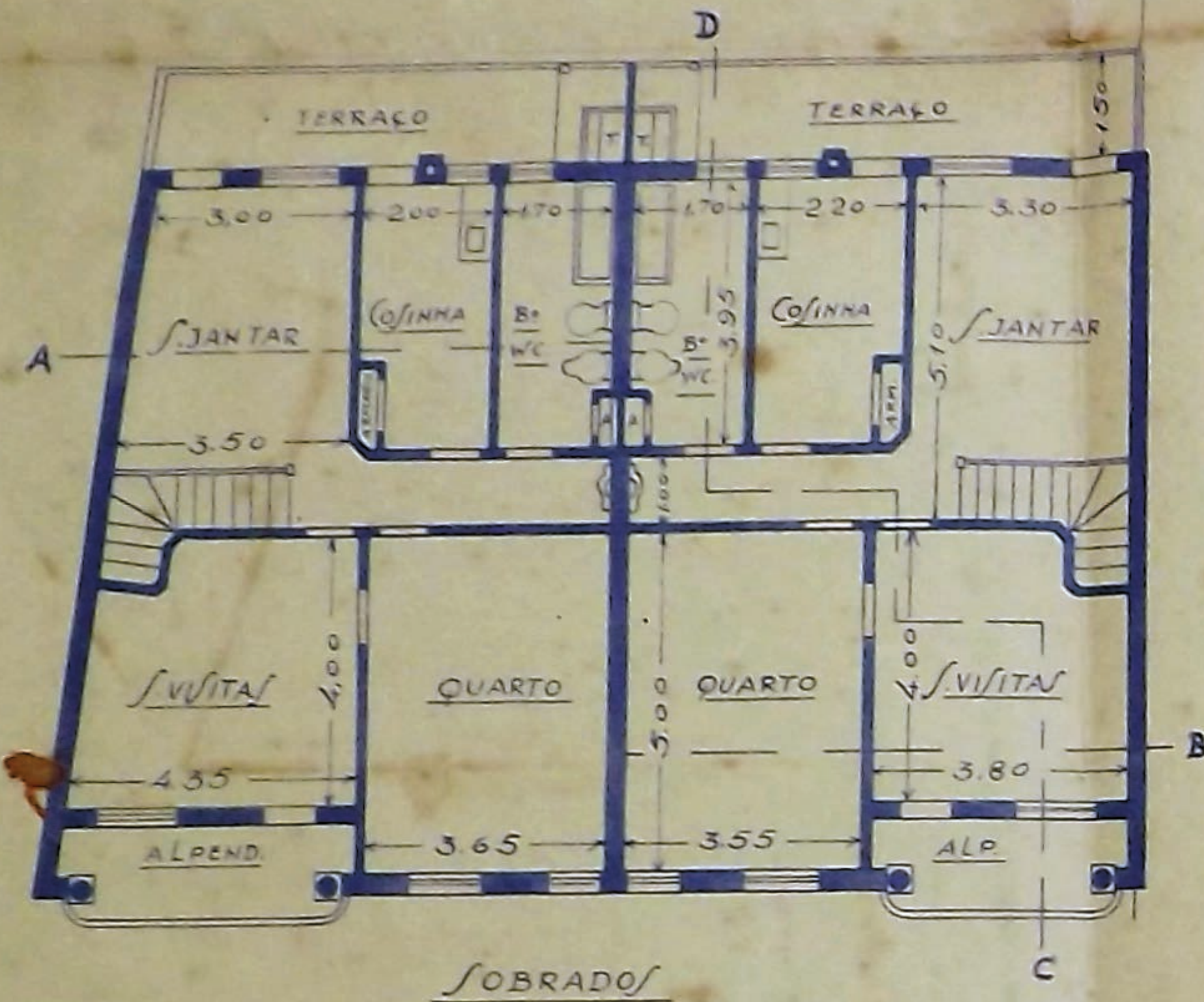
PLANTA - E/C 1:100
